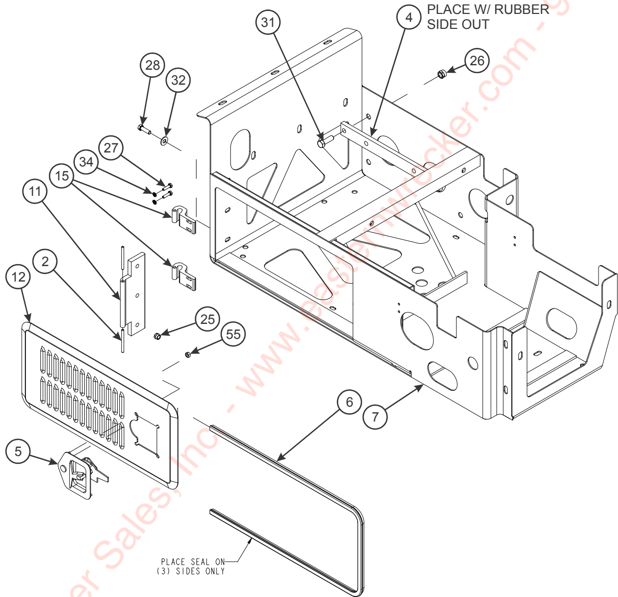
BASE - DOOR ASSEMBLY
